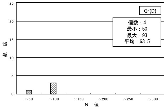
図 4.2.1 N 値の頻度分布図
