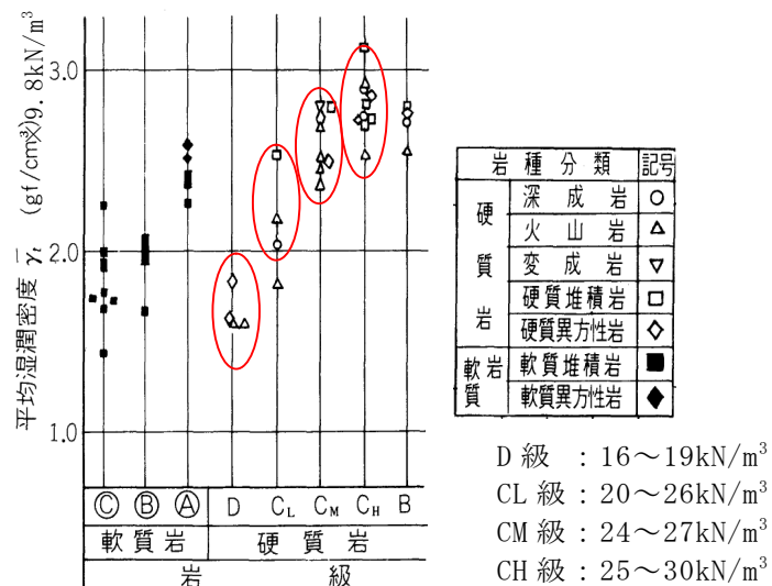
図 5.1.2 岩級区分と湿潤密度の一般的な関係
