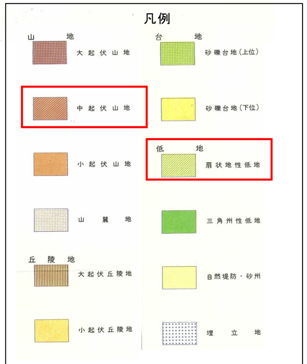
図 3.1.1 調査地周辺の地形分類図
