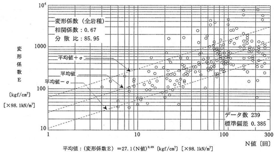
図 5.1.4 岩盤の変形係数の測定例（換算 N 値との関係）
