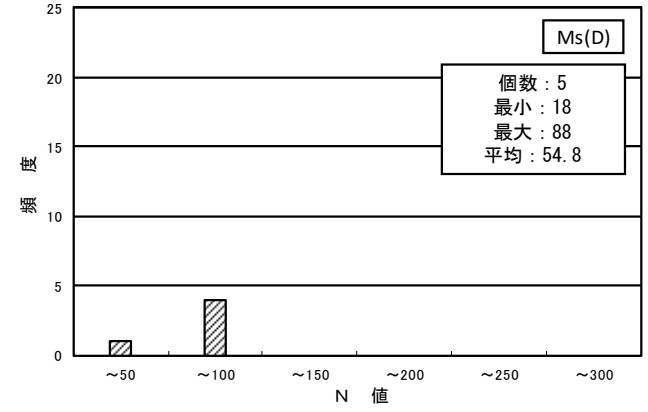
図 4.2.1 N 値の頻度分布図
